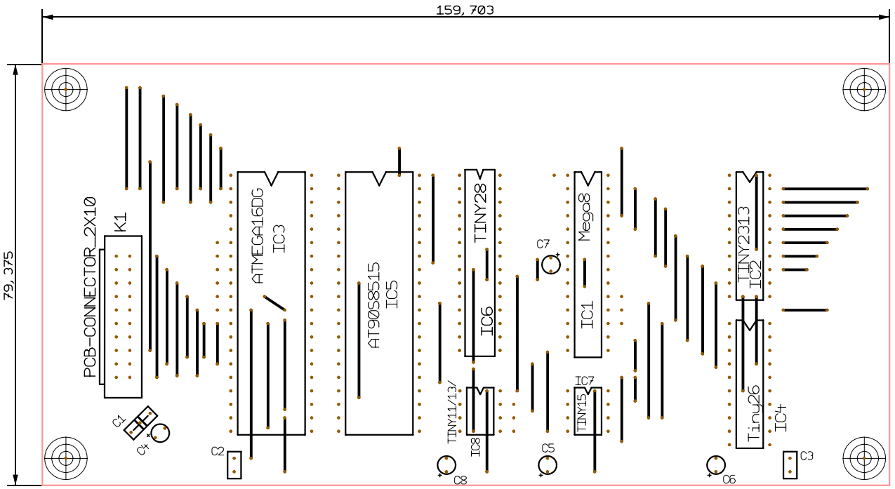
D. G. 0409 Adapter HV_Prog.
