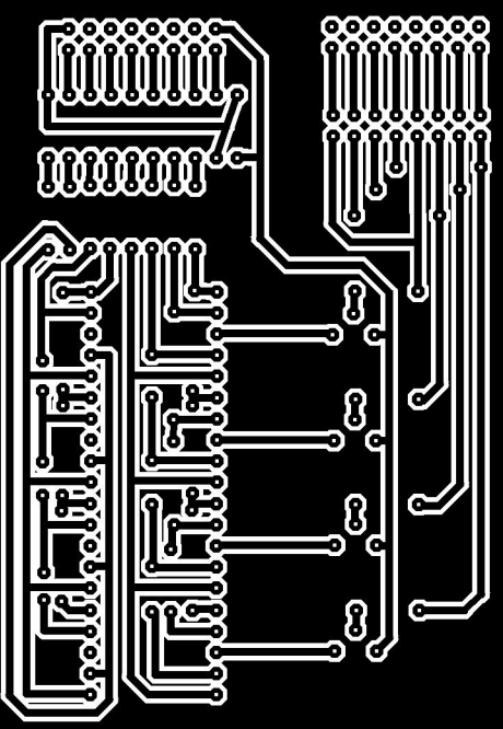
LED BOARD 4 FACH MULTIPLEX DATRONIX ANSCHLUSS
